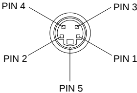
4 PIN MINI DIN FEMALE MATING FACE
